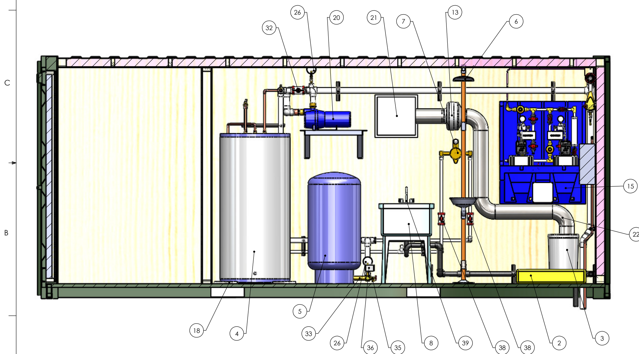
SECTION D-D SCALE 1 : 25
